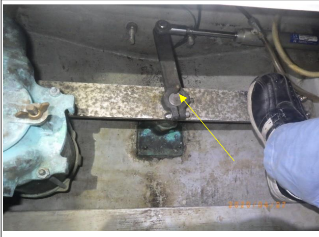
5 ラダー軸キー修正
